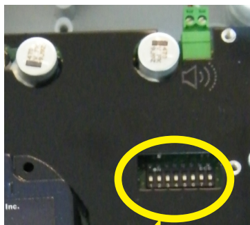
Dip-Schalterstellung
